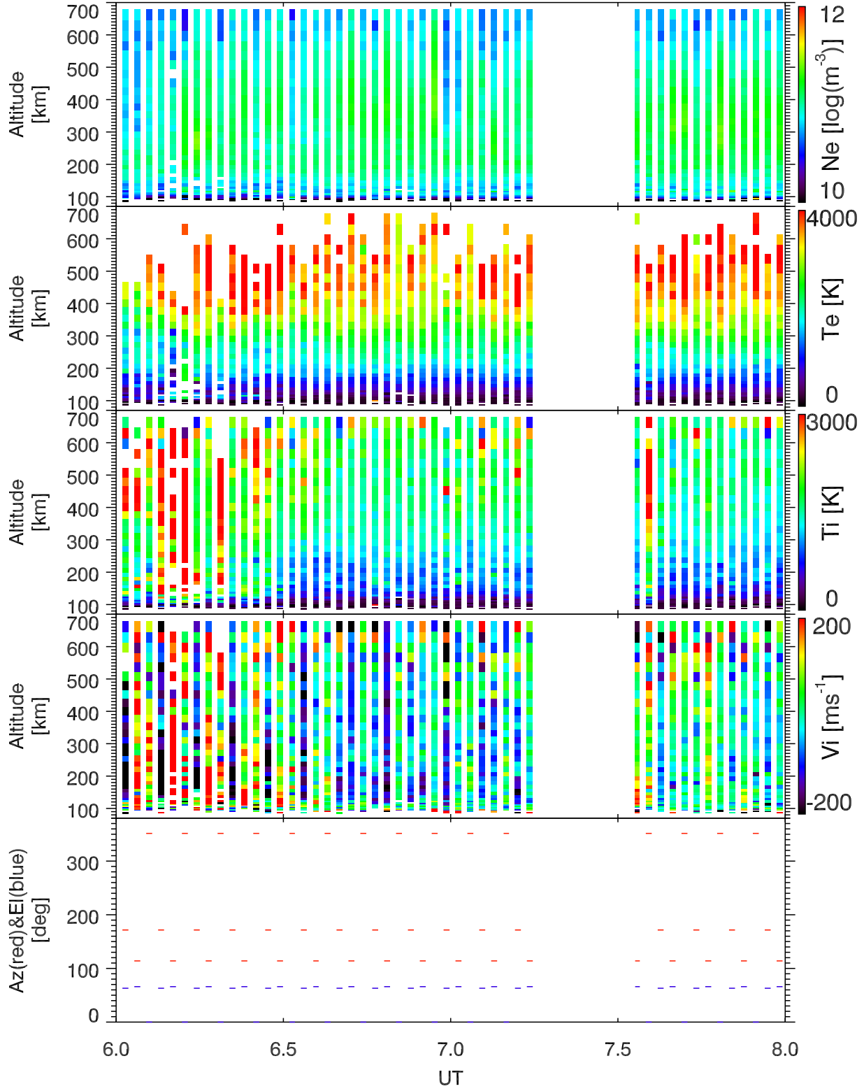
EISCAT 2002-08-01_06_08UT_tau0_ant@32m.
