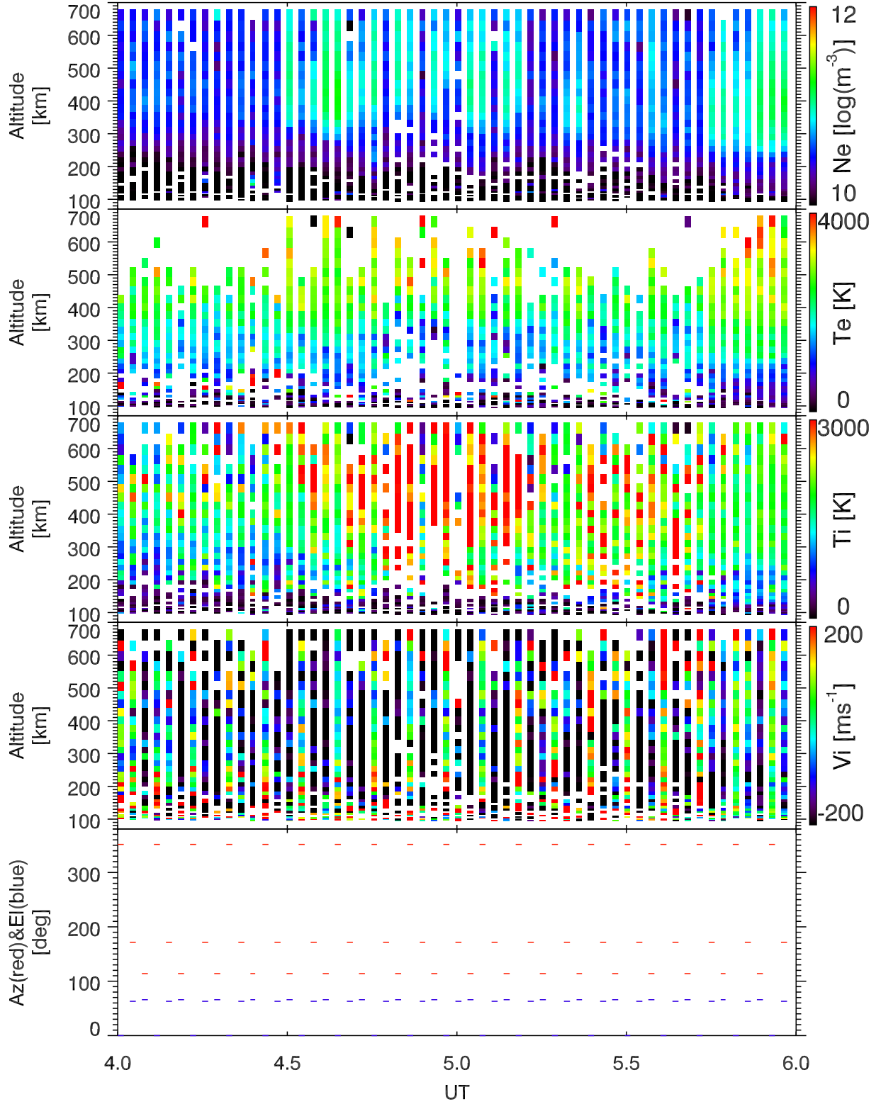
EISCAT 2002-10-10_04_06UT_tau0_ant@32m.
