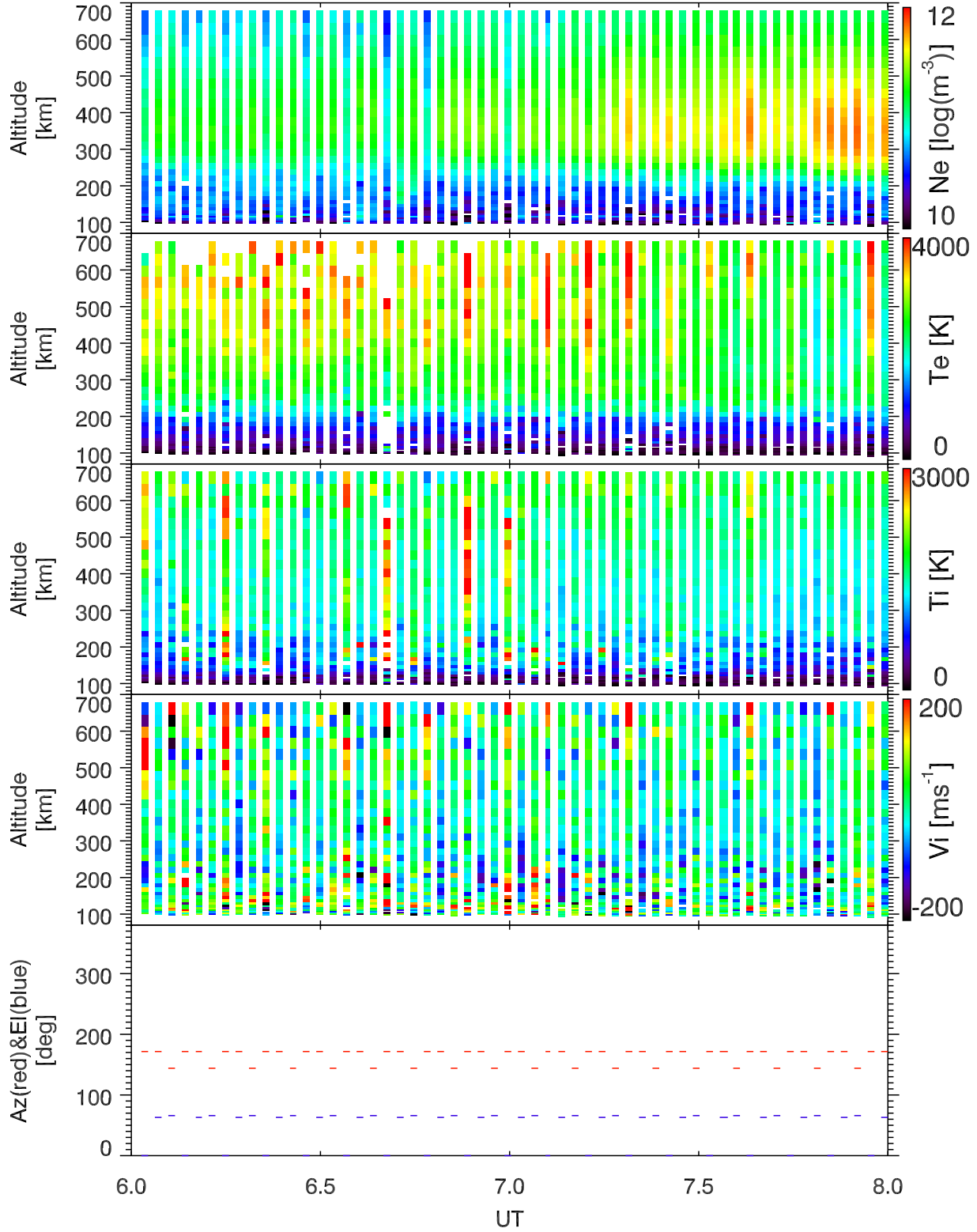
EISCAT 2002-10-11_06_08UT_tau0_ant@32m.
