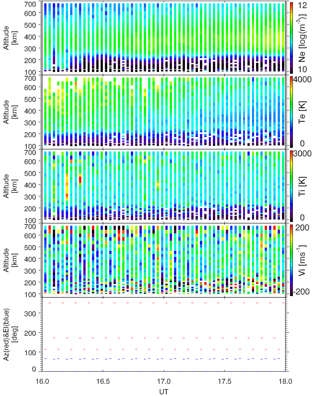
EISCAT 2002-10-12_16_18UT_tau0_ant@32m.
