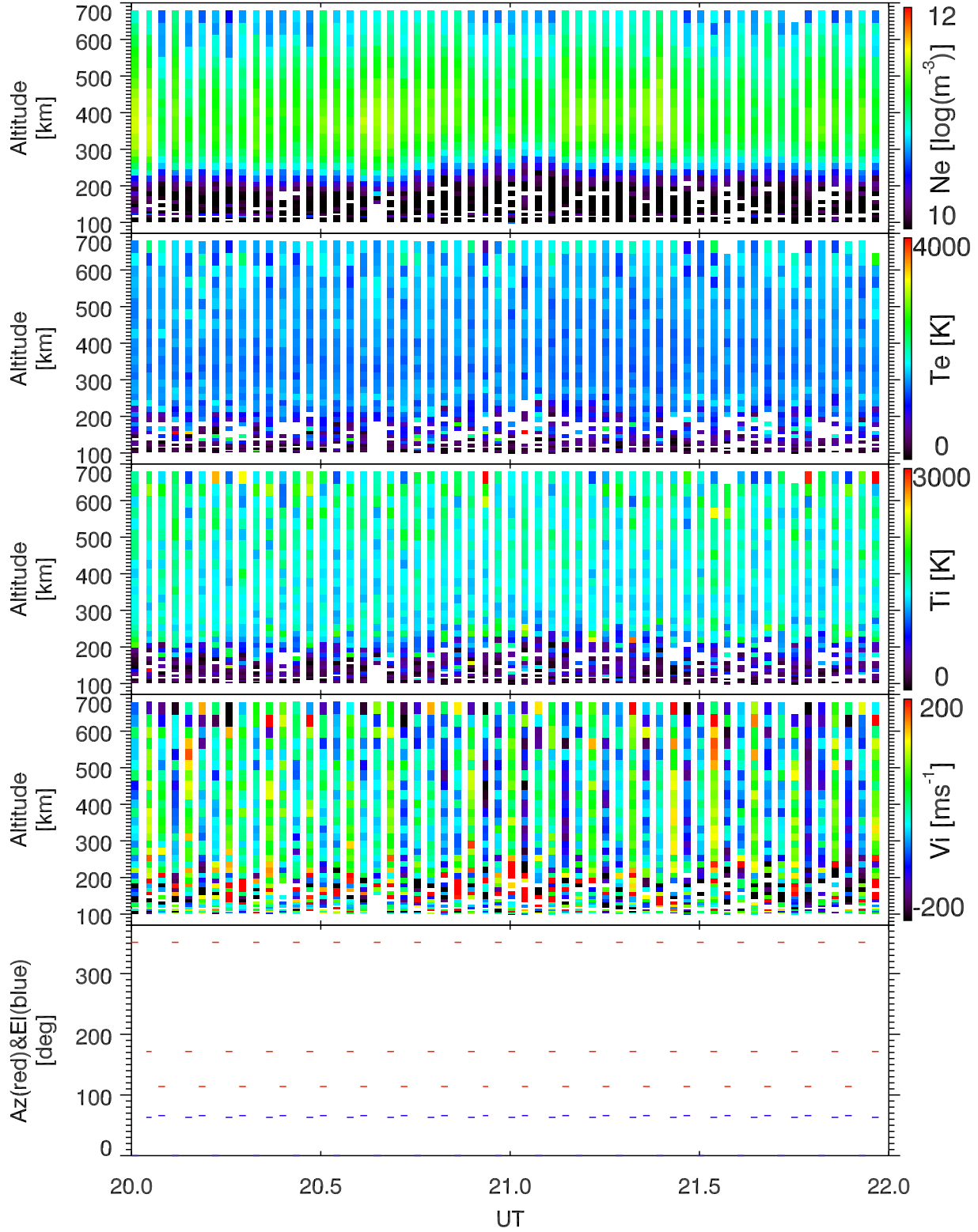
EISCAT 2002-10-12_20_22UT_tau0_ant@32m.
