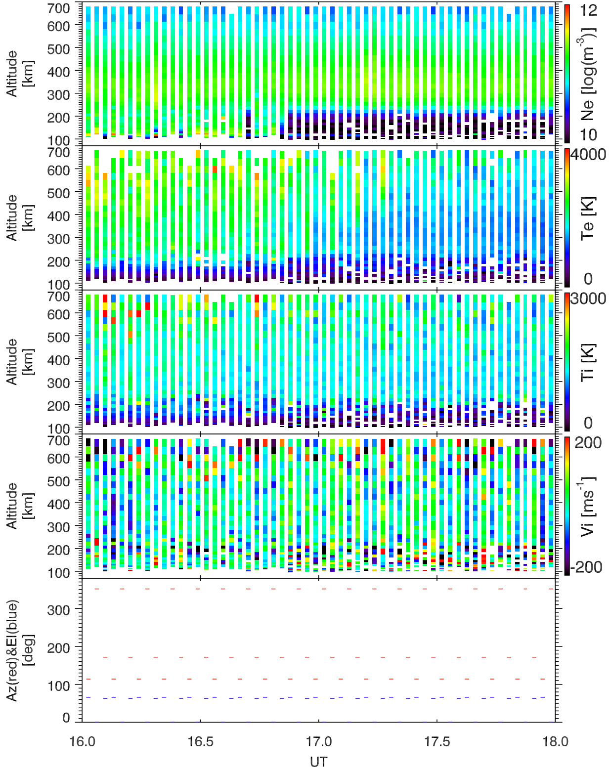
EISCAT 2002-10-13_16_18UT_tau0_ant@32m.
