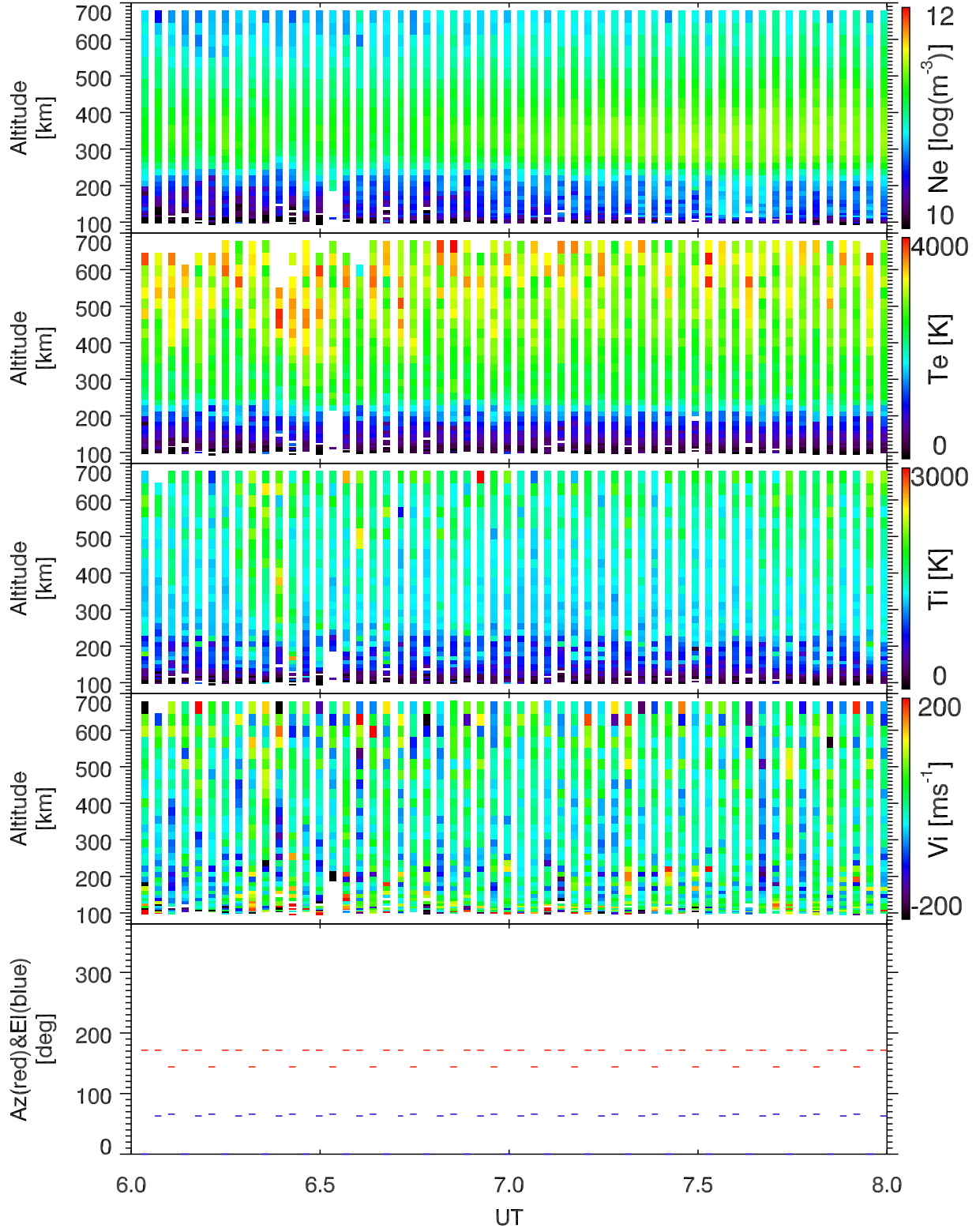
EISCAT 2002-10-16_06_08UT_tau0_ant@32m.
