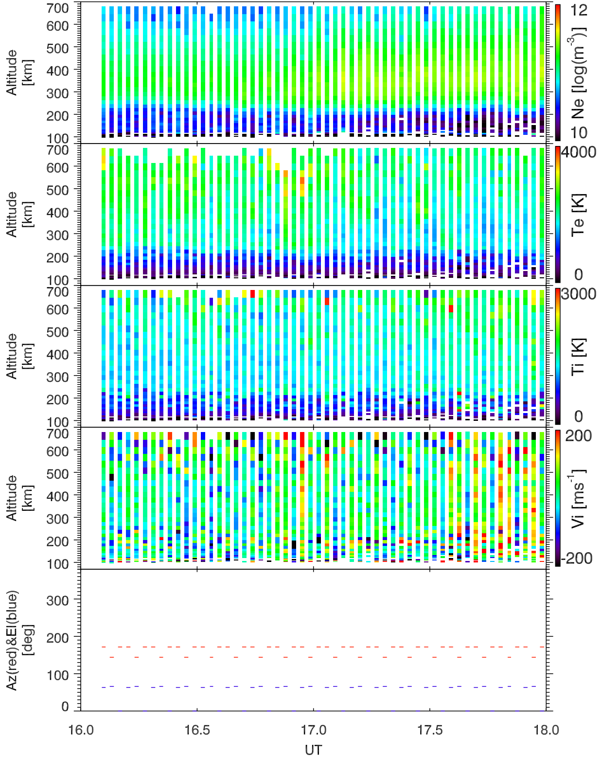
EISCAT 2002-10-16_16_18UT_tau0_ant@32m.
