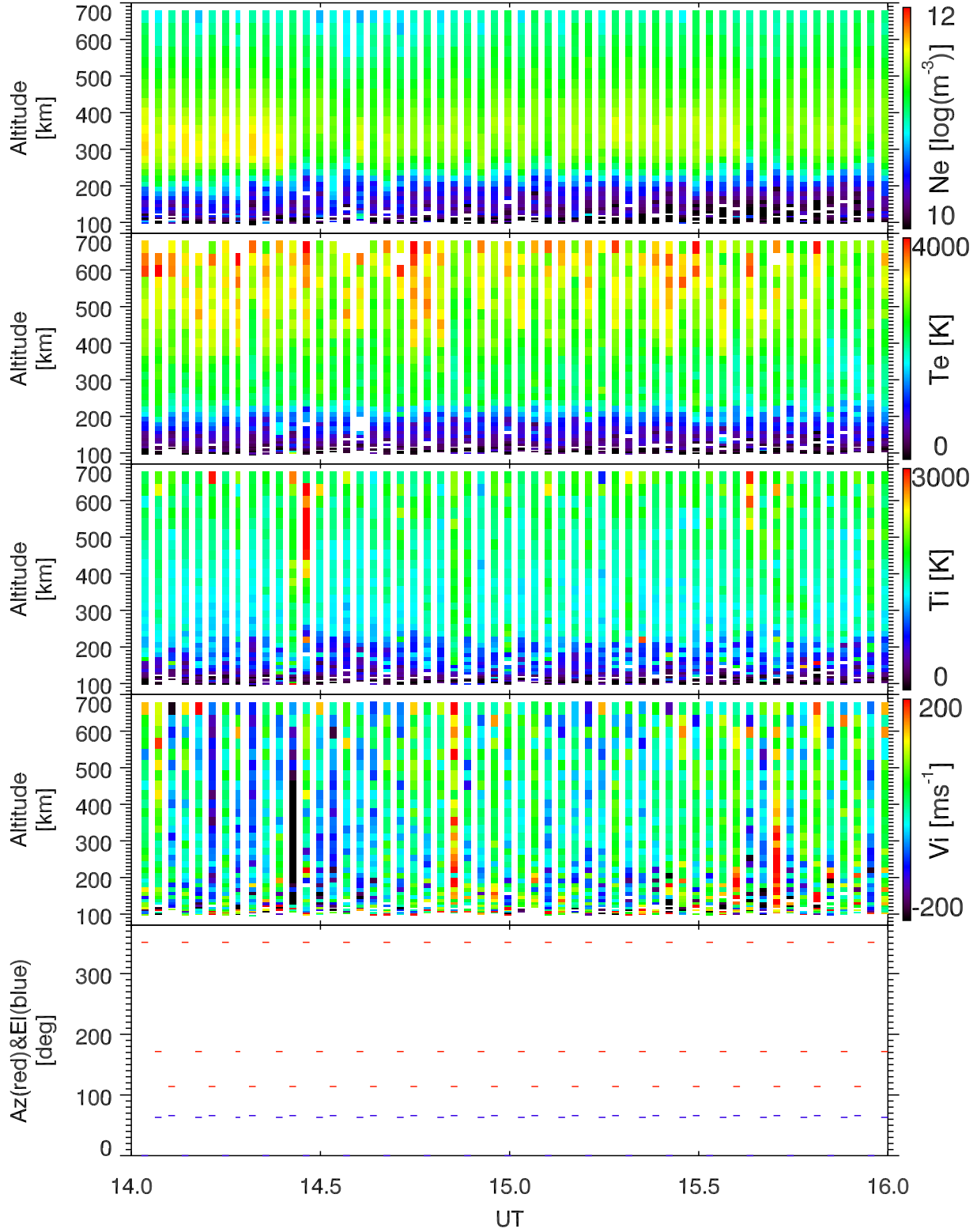
EISCAT 2002-10-17_14_16UT_tau0_ant@32m.
