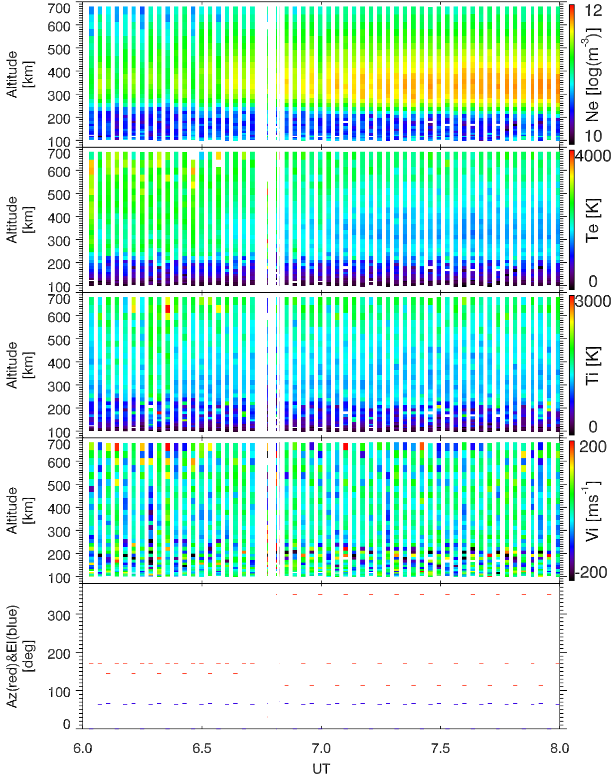
EISCAT 2002-10-20_06_08UT_tau0_ant@32m.
