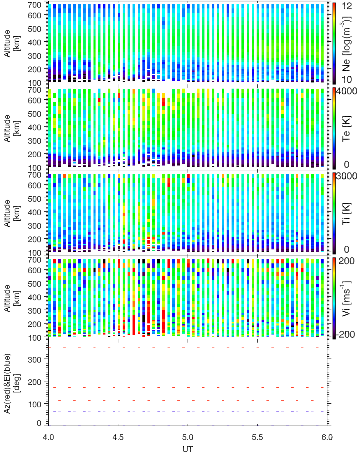
EISCAT 2002-10-22_04_06UT_tau0_ant@32m.
