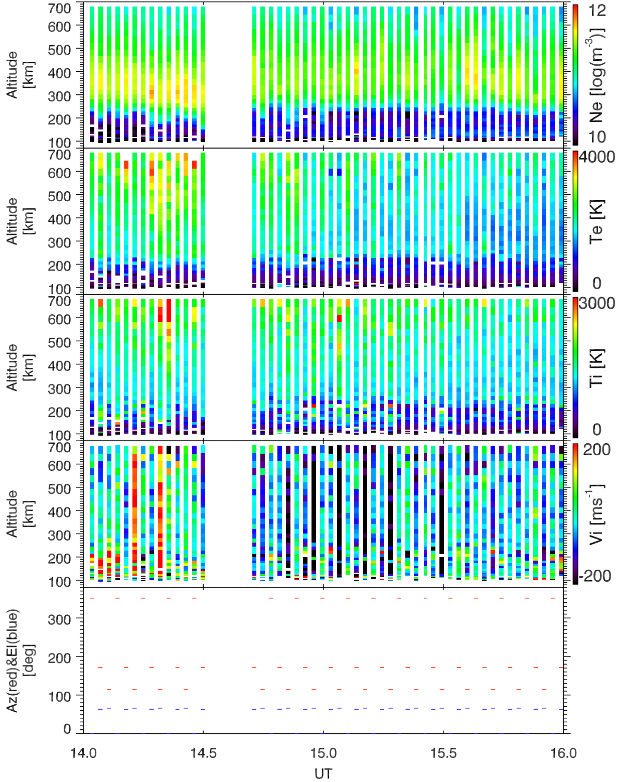
EISCAT 2002-10-22_14_16UT_tau0_ant@32m.
