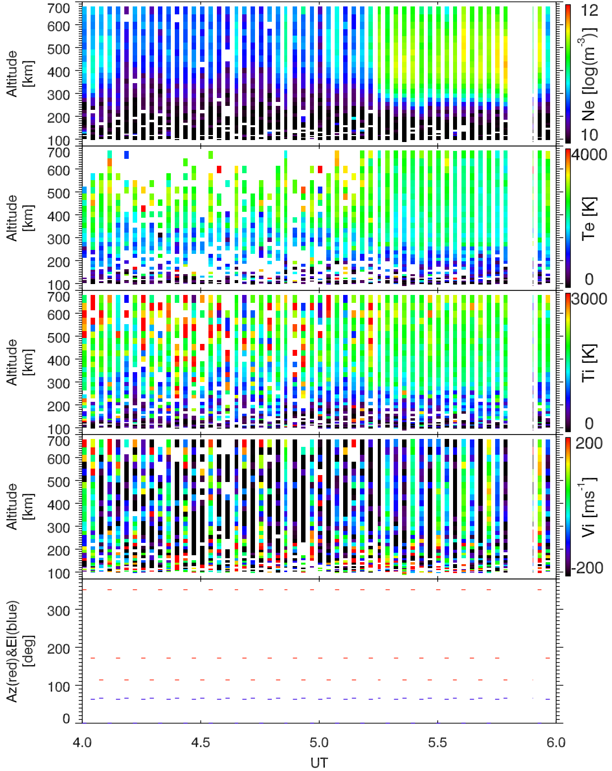
EISCAT 2002-10-24_04_06UT_tau0_ant@32m.
