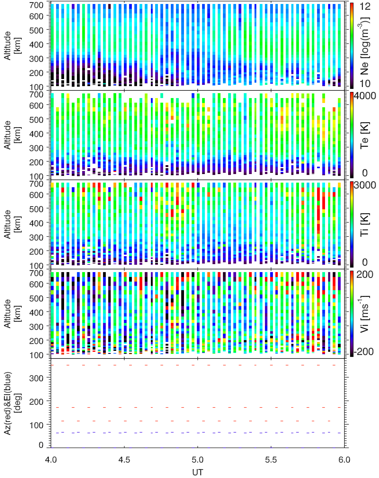
EISCAT 2002-10-26_04_06UT_tau0_ant@32m.
