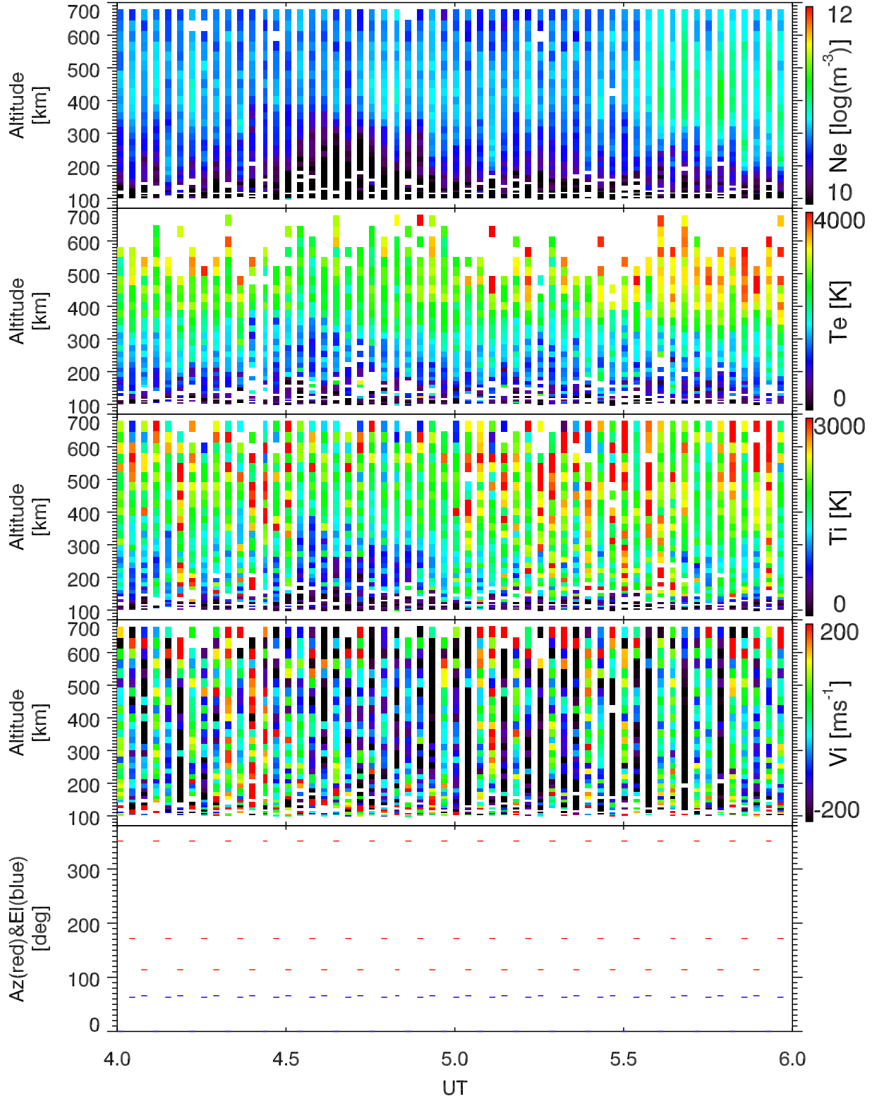
EISCAT 2002-10-28_04_06UT_tau0_ant@32m.
