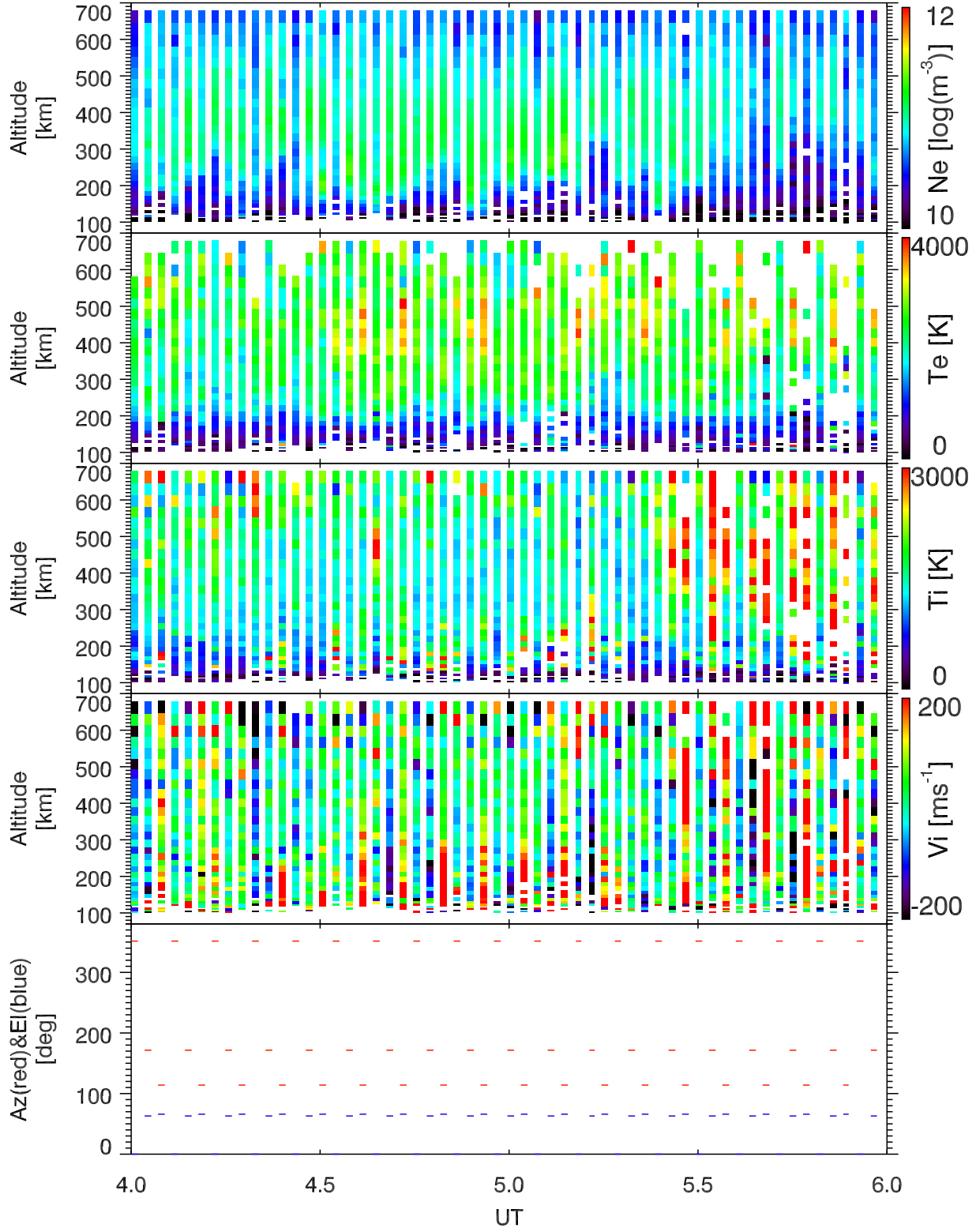
EISCAT 2002-10-30_04_06UT_tau0_ant@32m.
