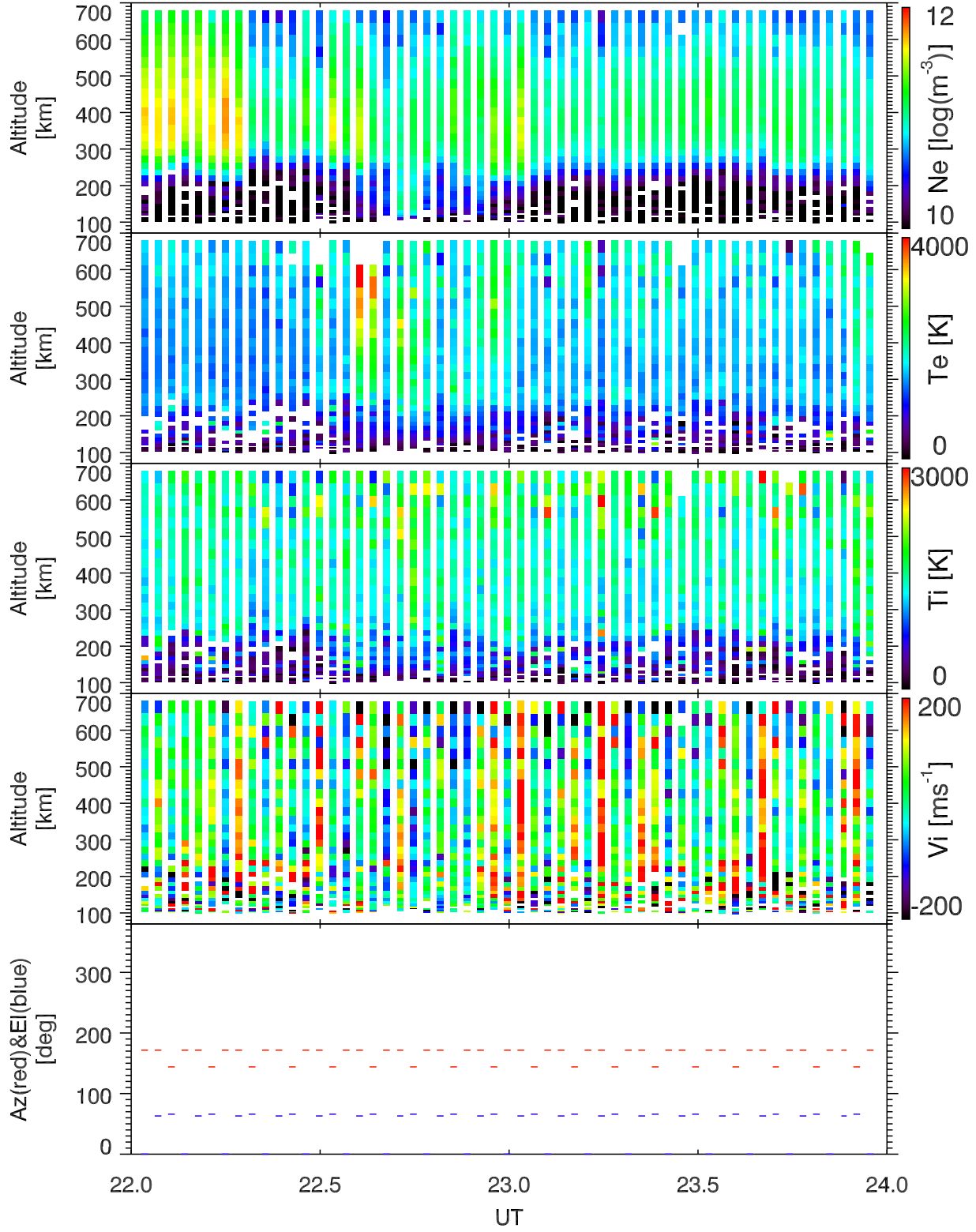
EISCAT 2002-10-30_22_24UT_tau0_ant@32m.
