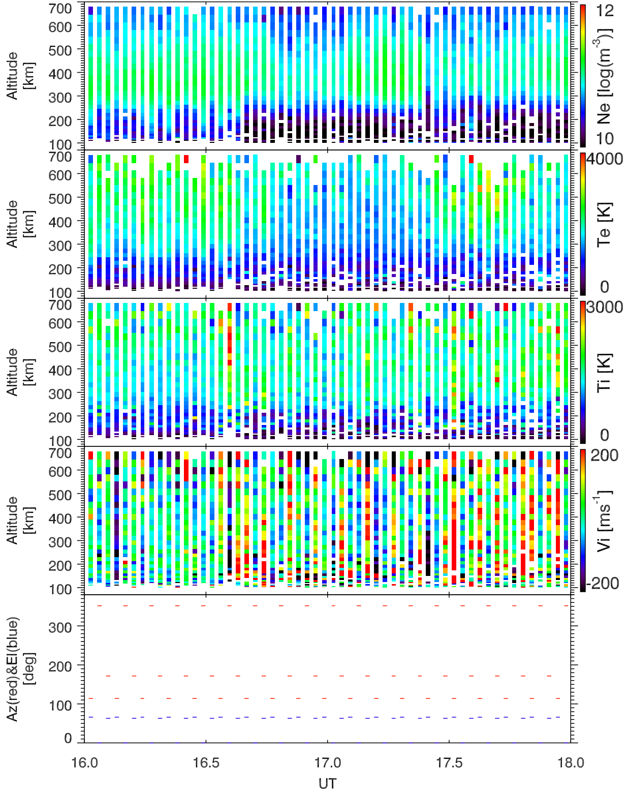
EISCAT 2002-11-02_16_18UT_tau0_ant@32m.
