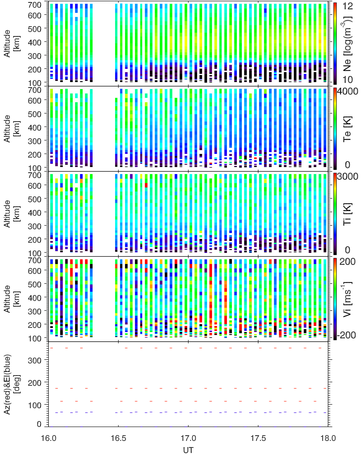
EISCAT 2002-11-12_16_18UT_tau0_ant@32m.
