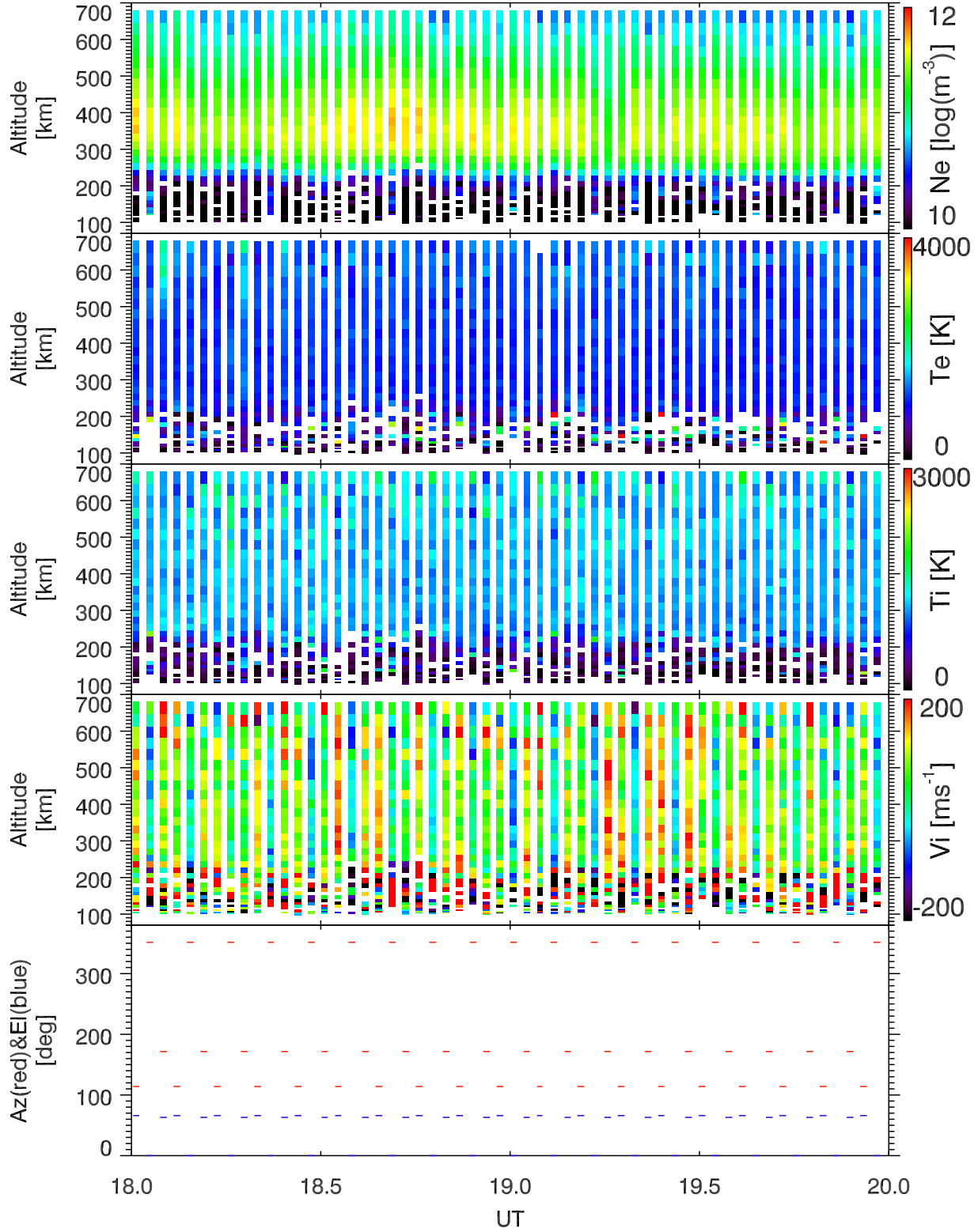
EISCAT 2002-11-13_18_20UT_tau0_ant@32m.
