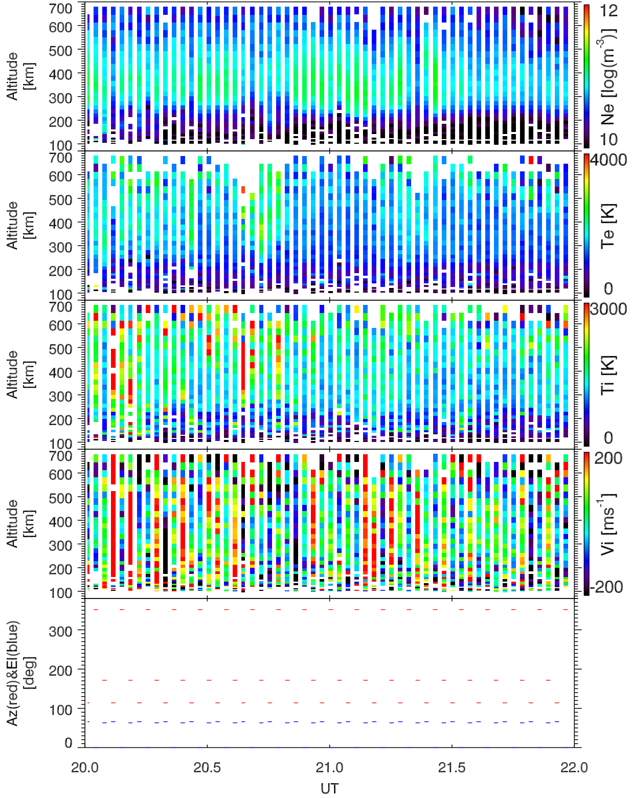
EISCAT 2003-02-17_20_22UT_tau0_ant@32m.
