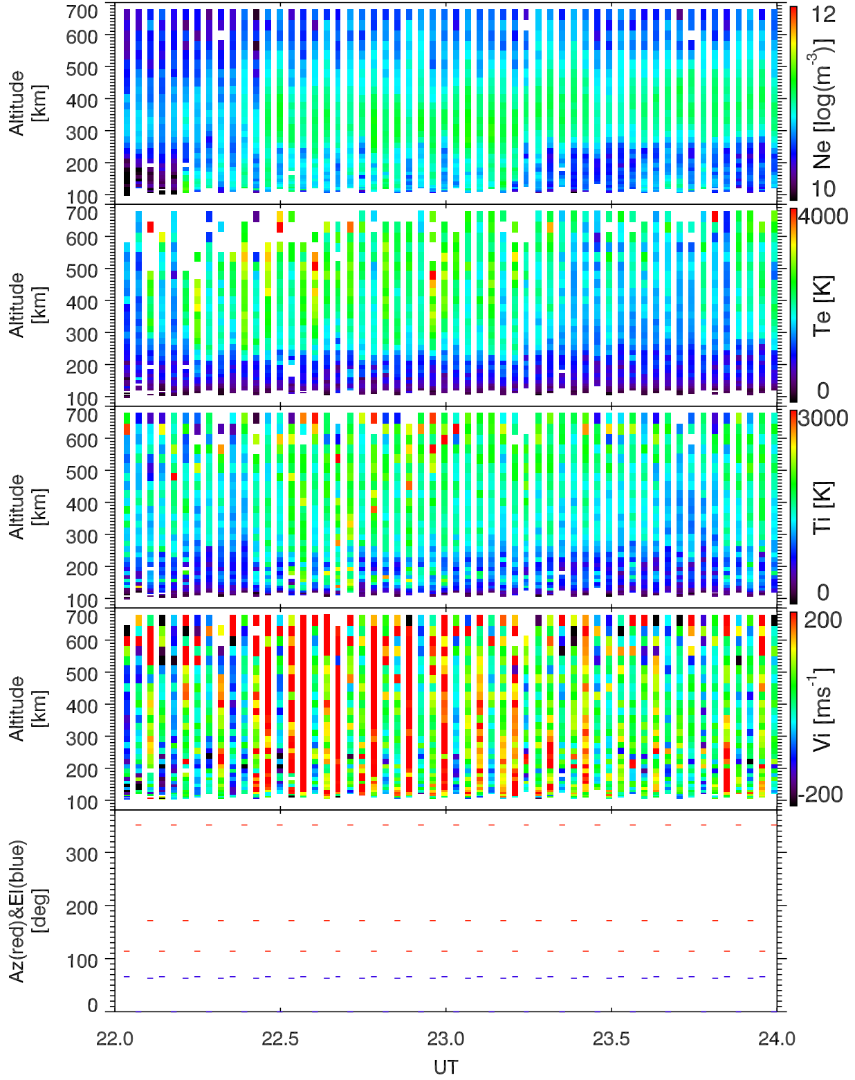
EISCAT 2003-02-17_22_24UT_tau0_ant@32m.
