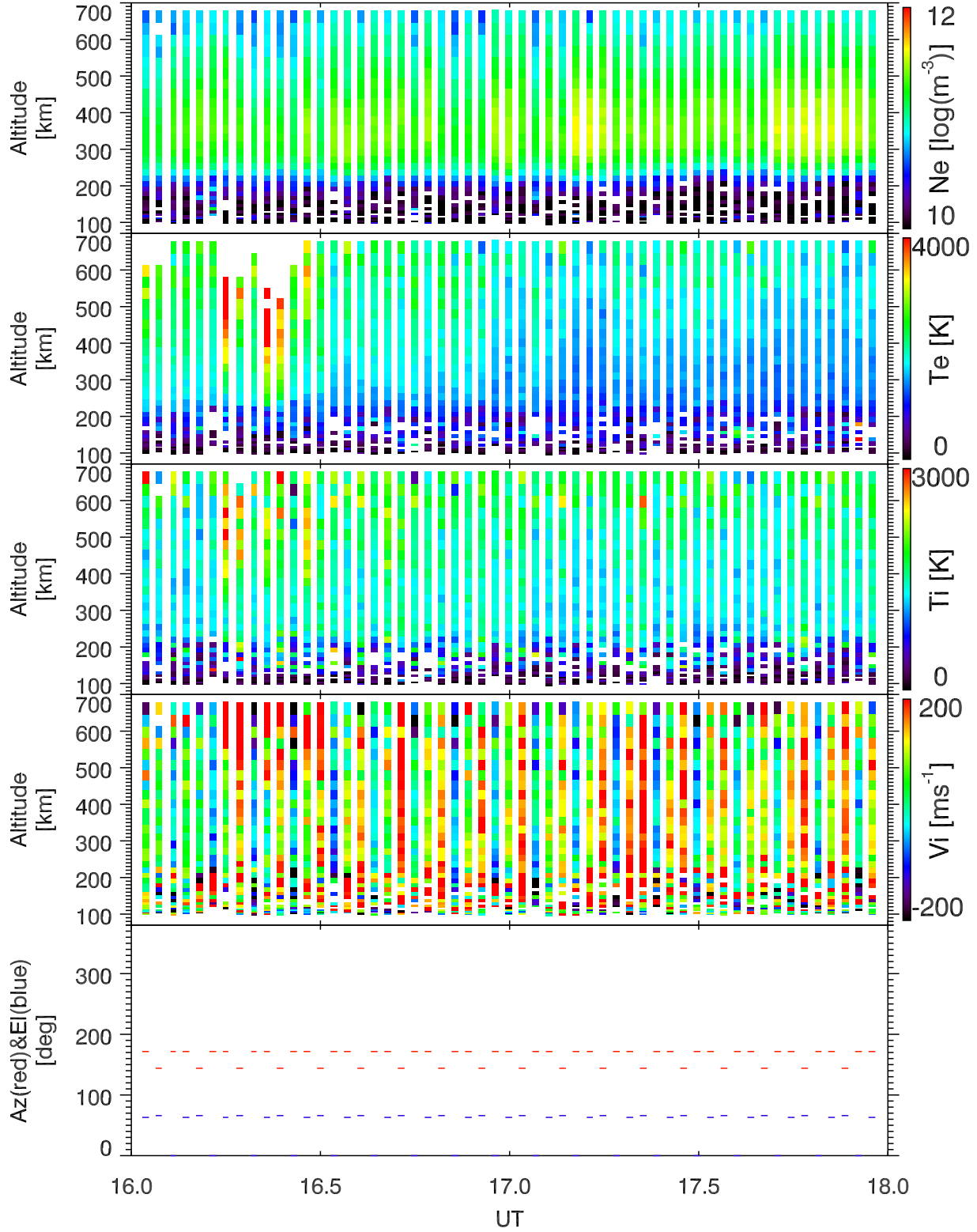
EISCAT 2003-02-28_16_18UT_tau0_ant@32m.
