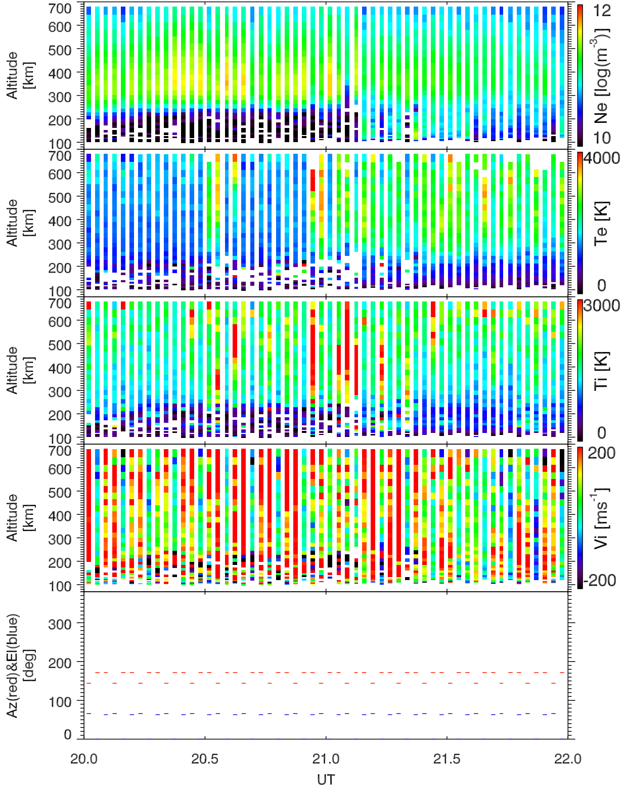
EISCAT 2003-02-28_20_22UT_tau0_ant@32m.
