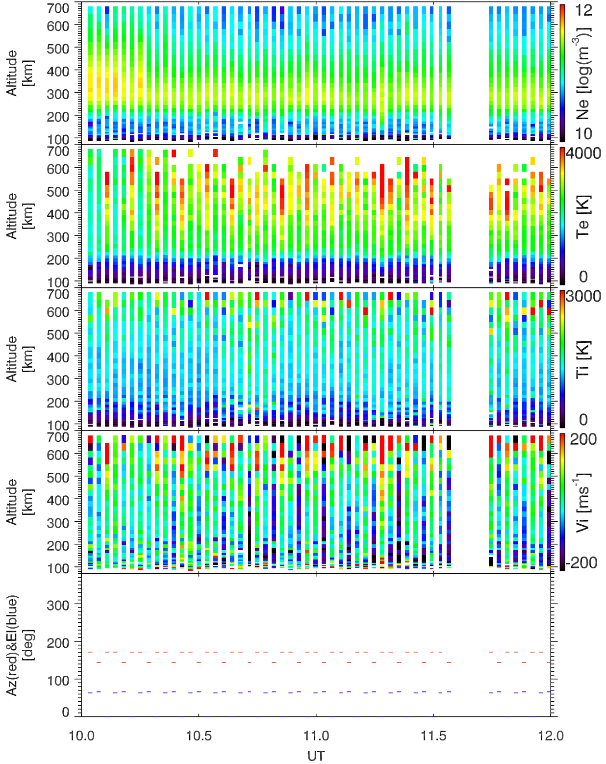
EISCAT 2003-03-03_10_12UT_tau0_ant@32m.
