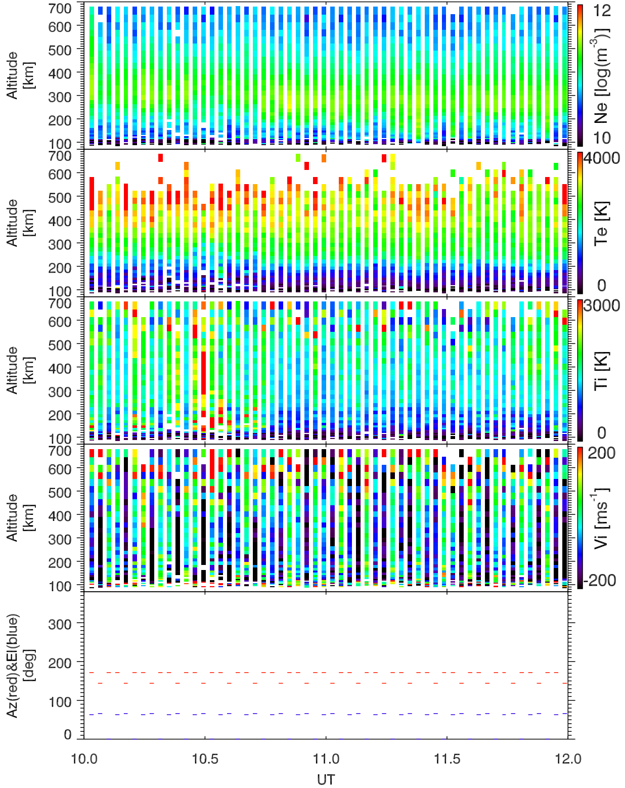
EISCAT 2003-03-15_10_12UT_tau0_ant@32m.
