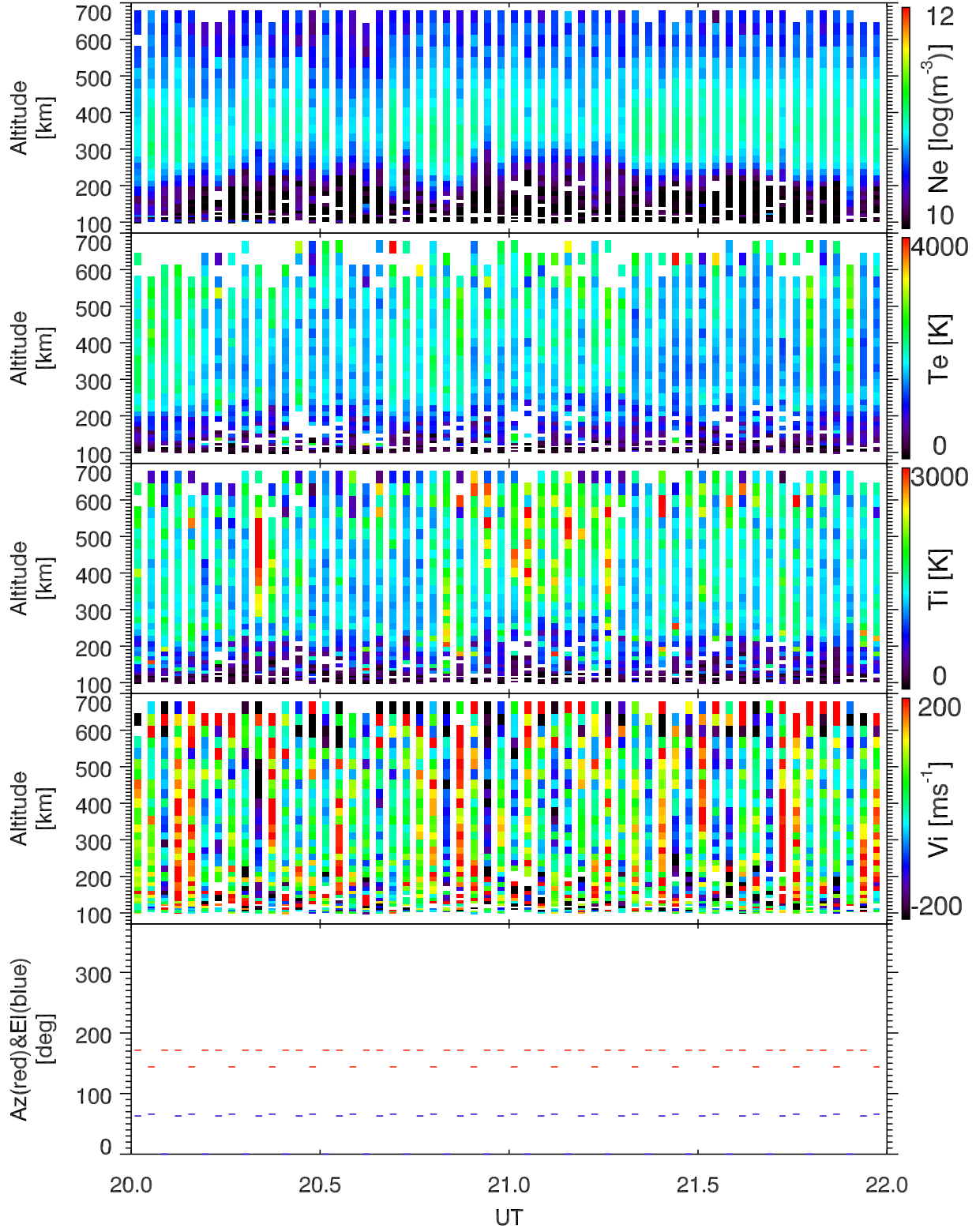
EISCAT 2003-03-19_20_22UT_tau0_ant@32m.
