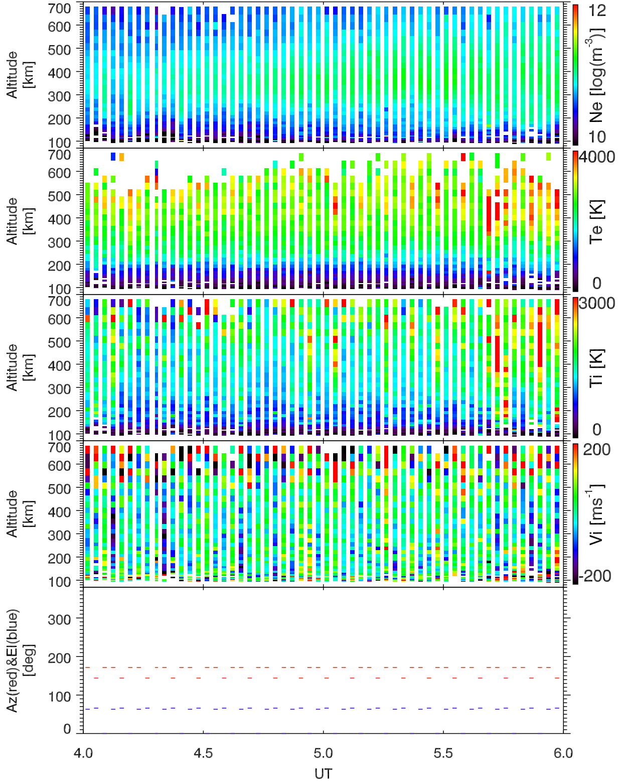
EISCAT 2003-03-20_04_06UT_tau0_ant@32m.
