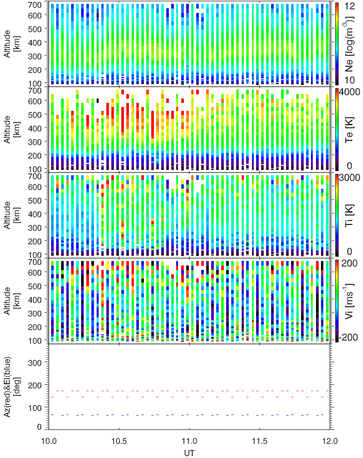
EISCAT 2003-03-20_10_12UT_tau0_ant@32m.
