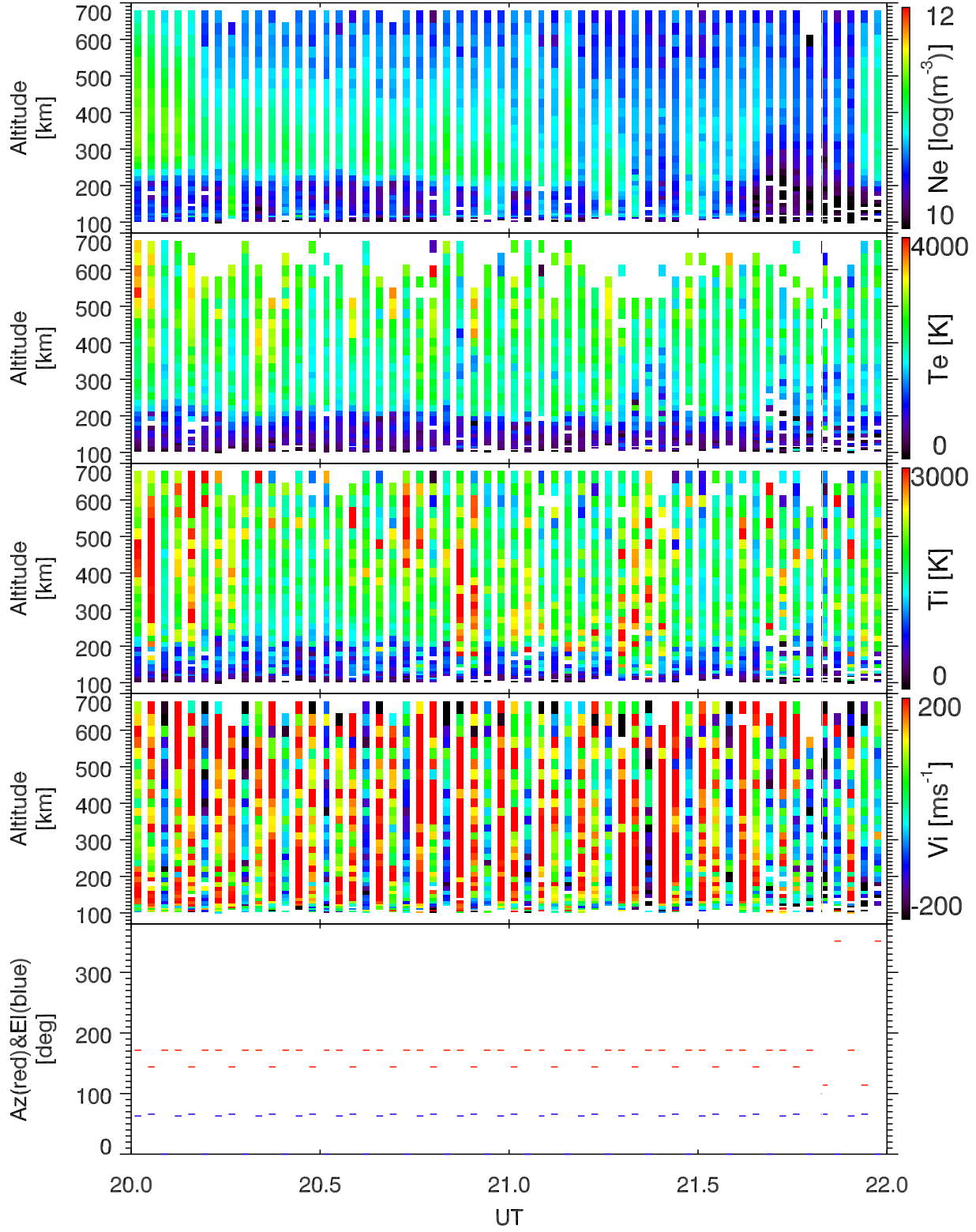
EISCAT 2003-03-20_20_22UT_tau0_ant@32m.
