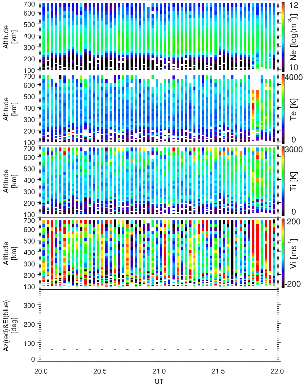
EISCAT 2003-03-21_20_22UT_tau0_ant@32m.
