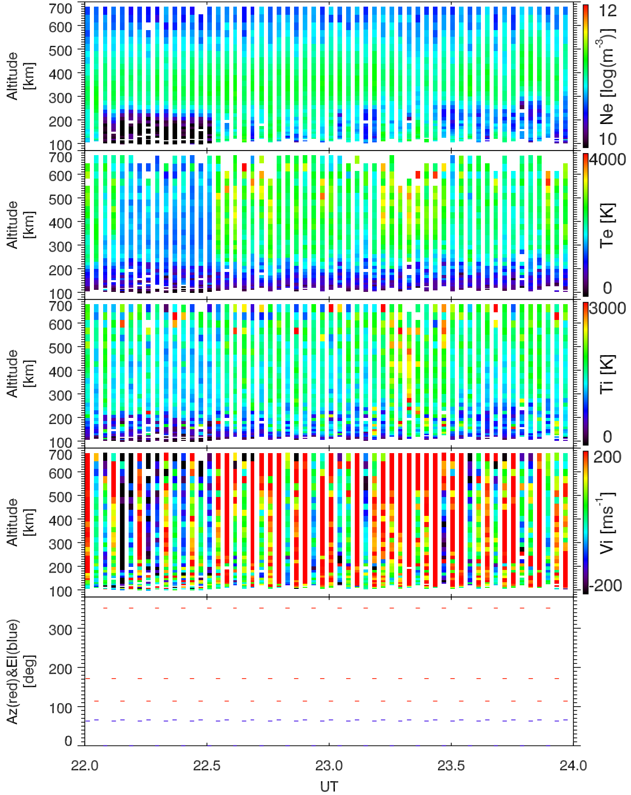
EISCAT 2003-03-21_22_24UT_tau0_ant@32m.
