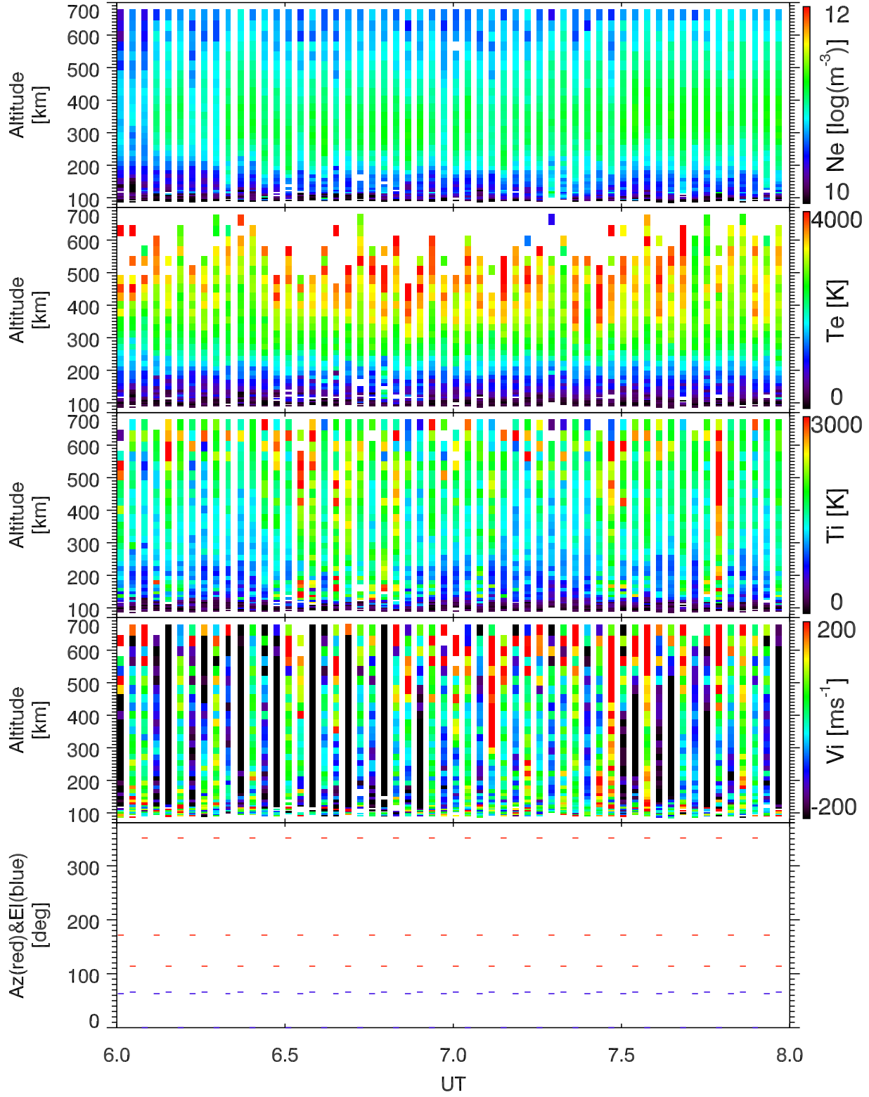
EISCAT 2003-03-22_06_08UT_tau0_ant@32m.
