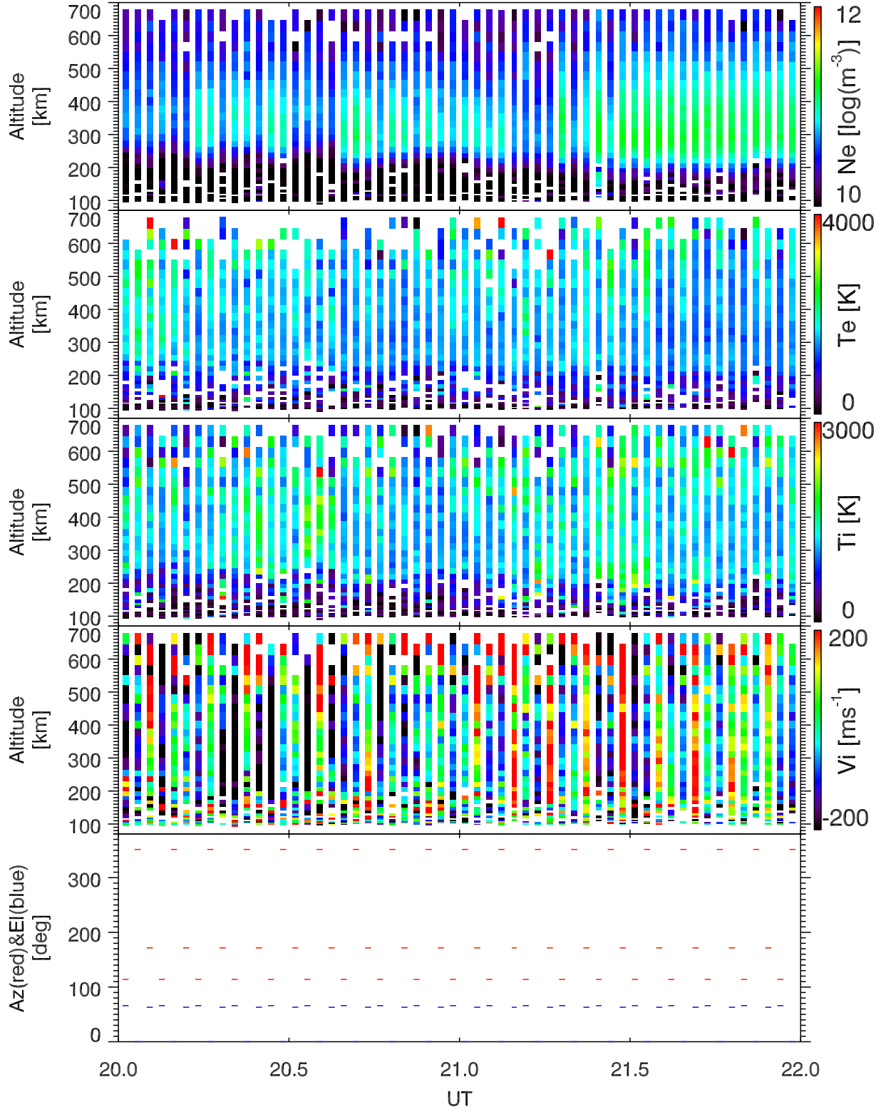
EISCAT 2003-03-22_20_22UT_tau0_ant@32m.
