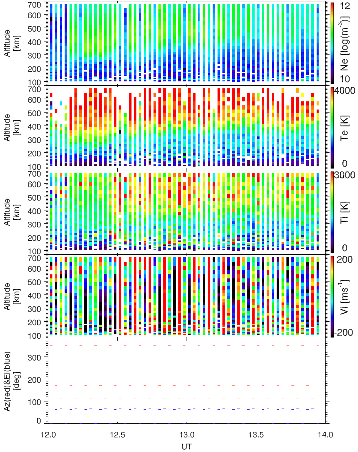
EISCAT 2003-10-29_12_14UT_tau0_ant@32m.
