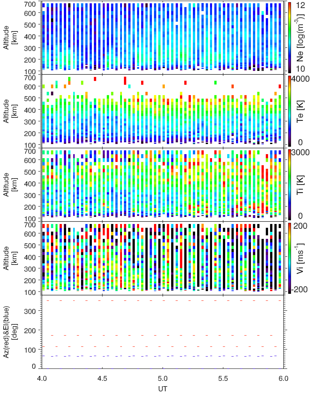
EISCAT 2003-10-30_04_06UT_tau0_ant@32m.
