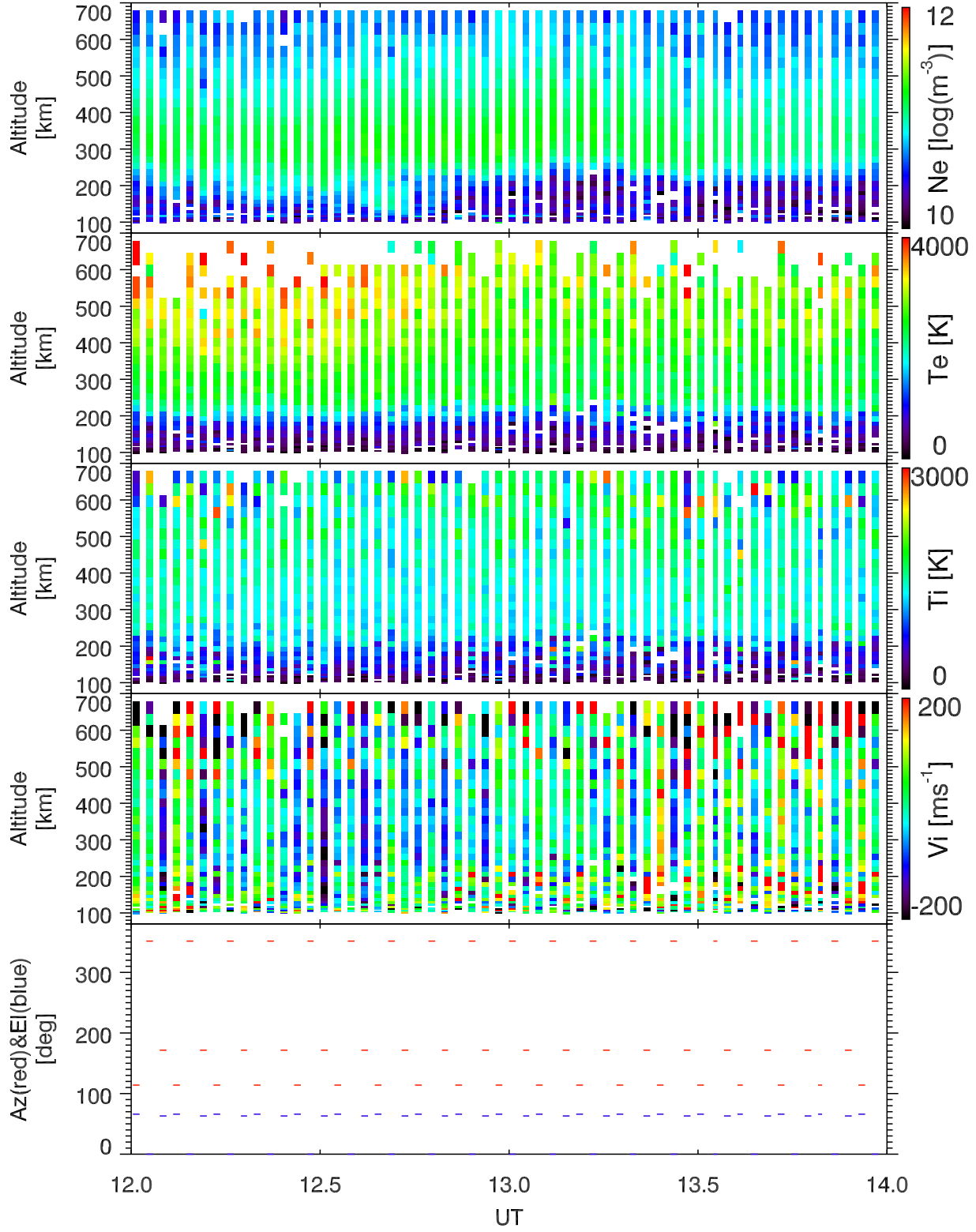
EISCAT 2003-10-30_12_14UT_tau0_ant@32m.
