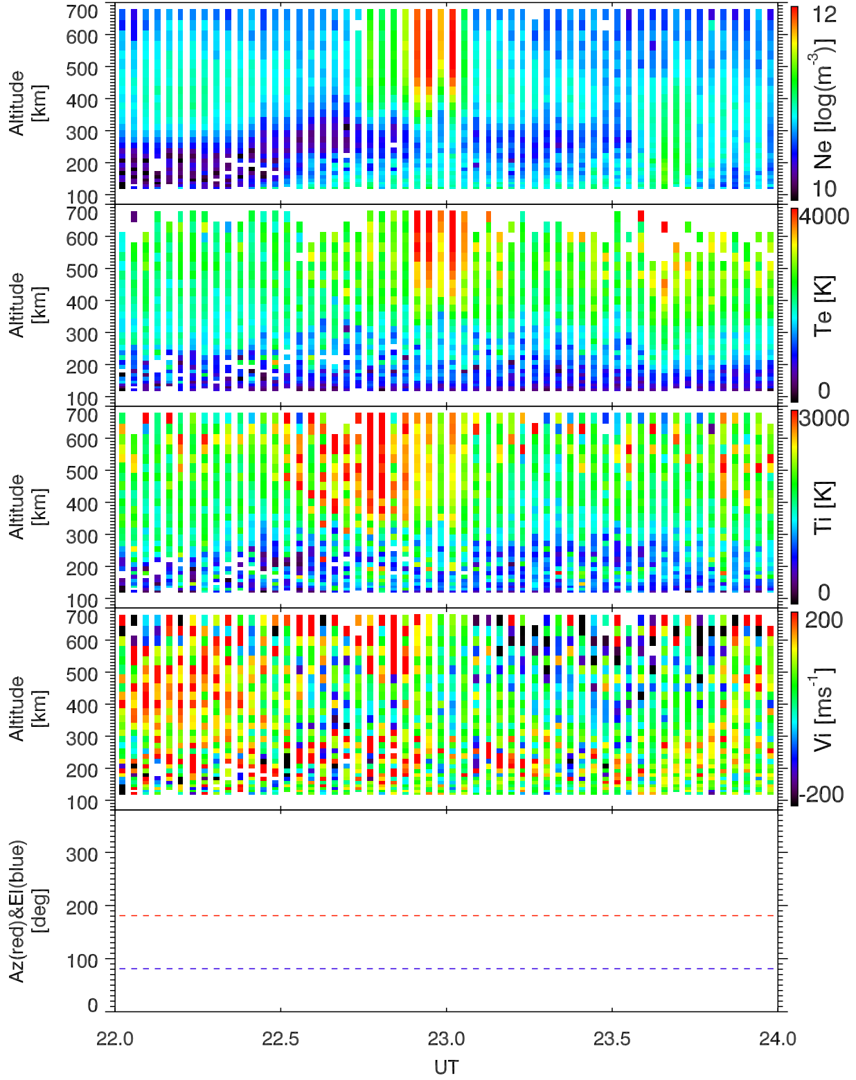
EISCAT 2003-10-30_22_24UT_tau0_ant@42m.
