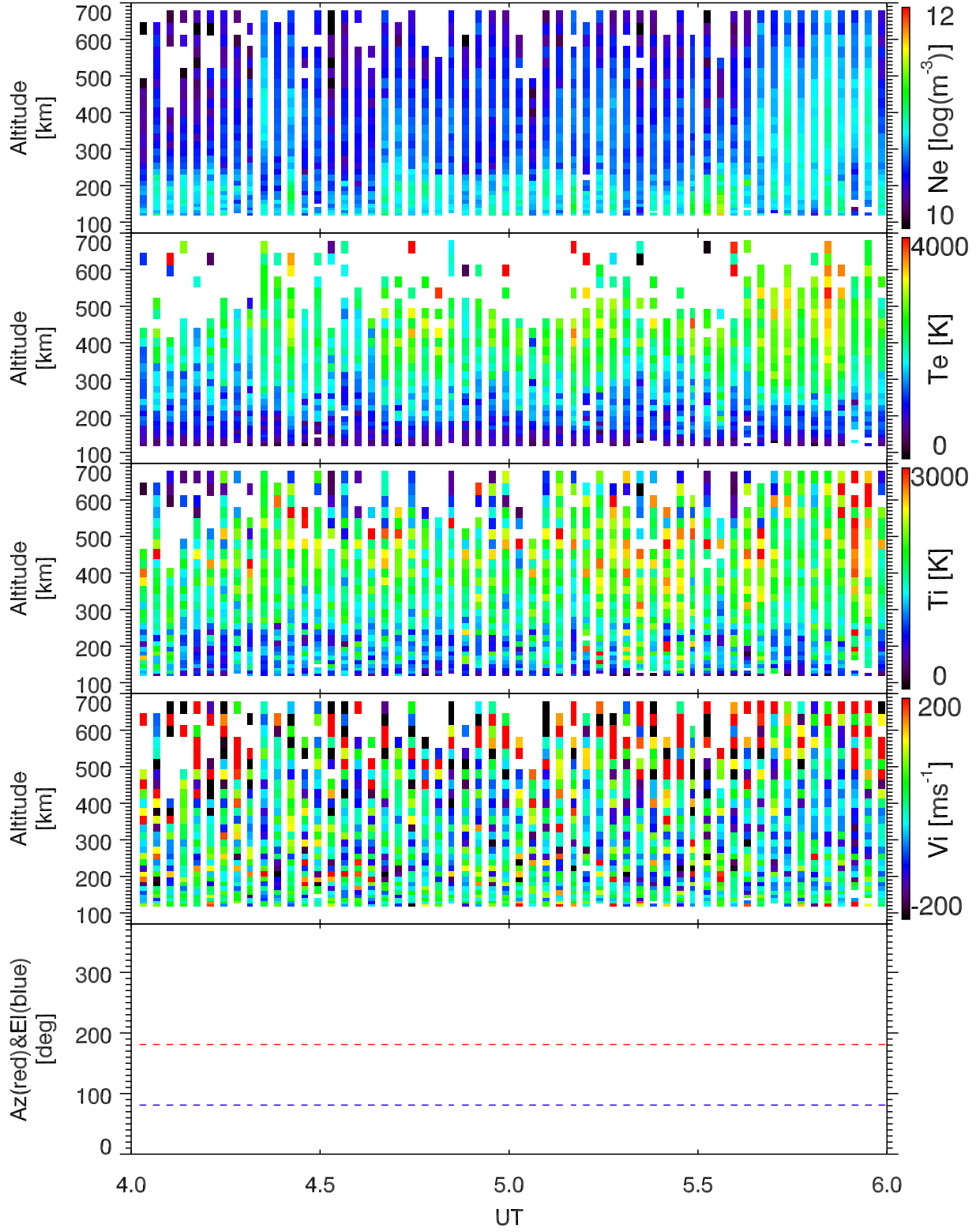
EISCAT 2003-11-01_04_06UT_tau0_ant@42m.
