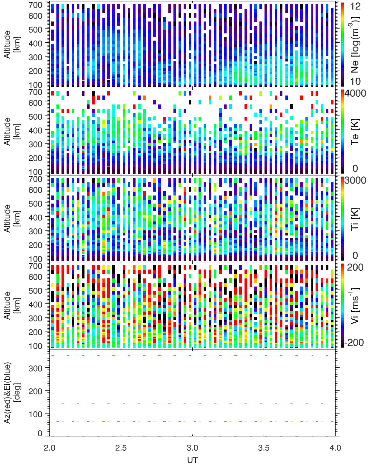
EISCAT 2003-11-12_02_04UT_steffe_ant@32m.
