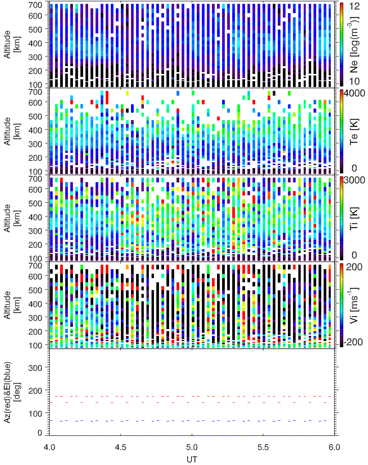
EISCAT 2003-11-14_04_06UT_steffe_ant@32m.
