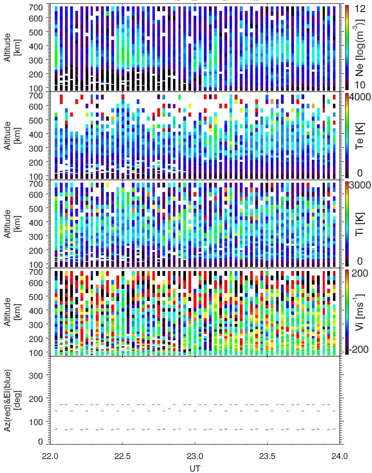
EISCAT 2003-11-14_22_24UT_steffe_ant@32m.
