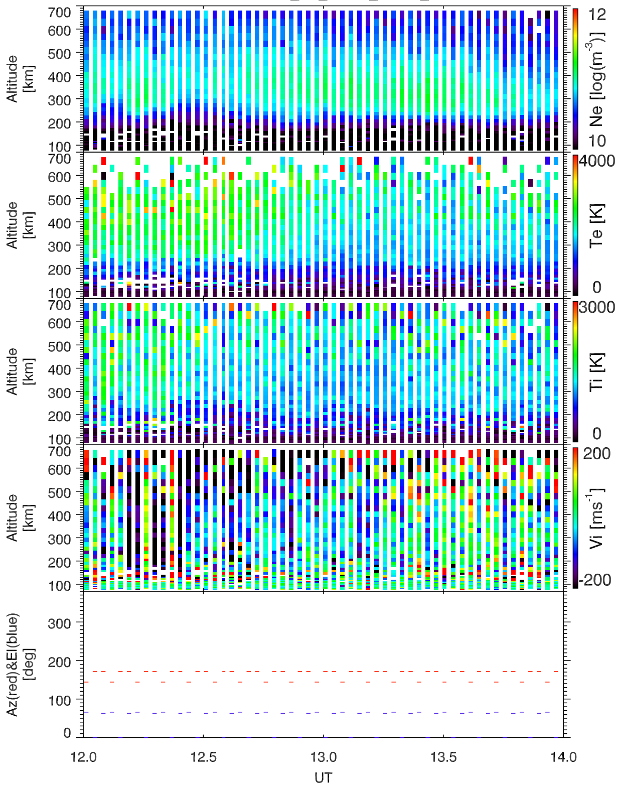
EISCAT 2003-11-15_12_14UT_steffe_ant@32m.
