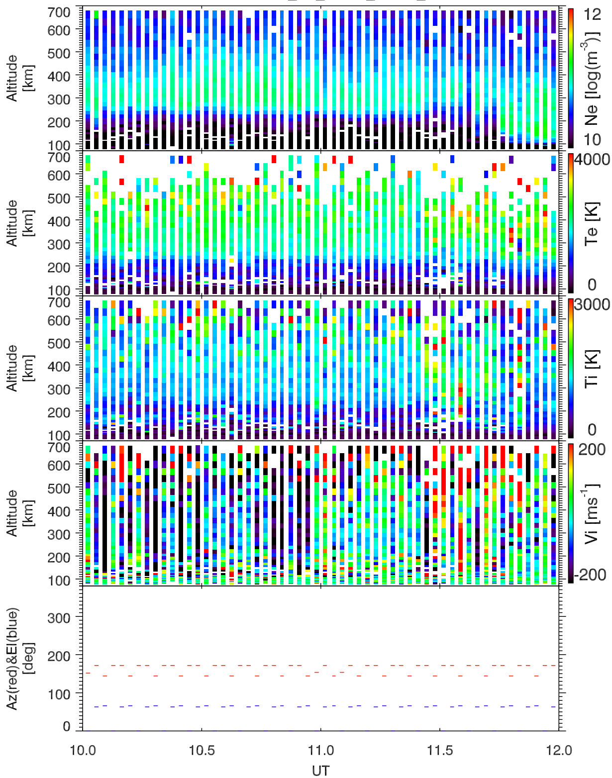
EISCAT 2003-11-17_10_12UT_steffe_ant@32m.
