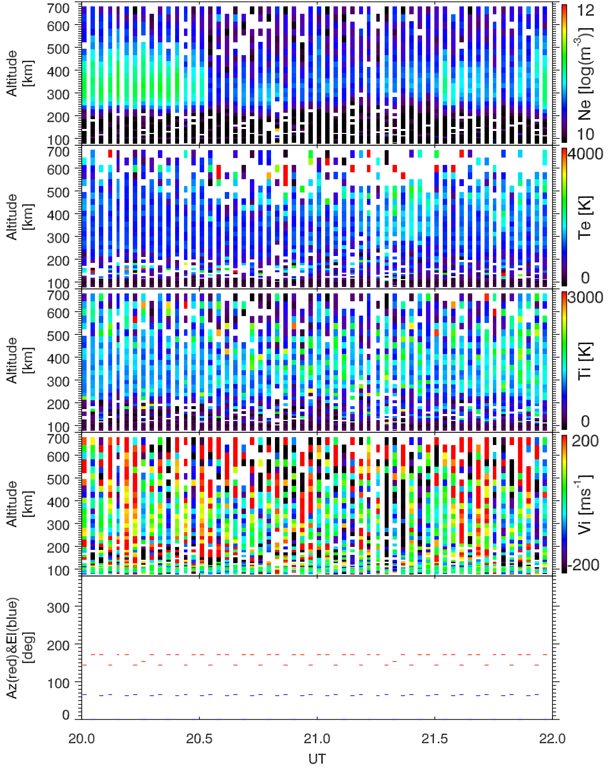
EISCAT 2003-11-17_20_22UT_steffe_ant@32m.
