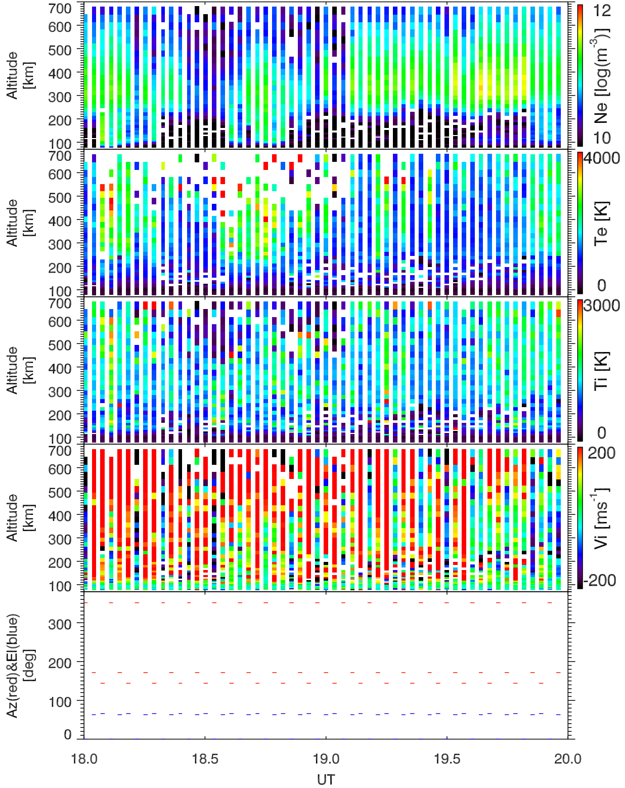
EISCAT 2003-11-18_18_20UT_steffe_ant@32m.
