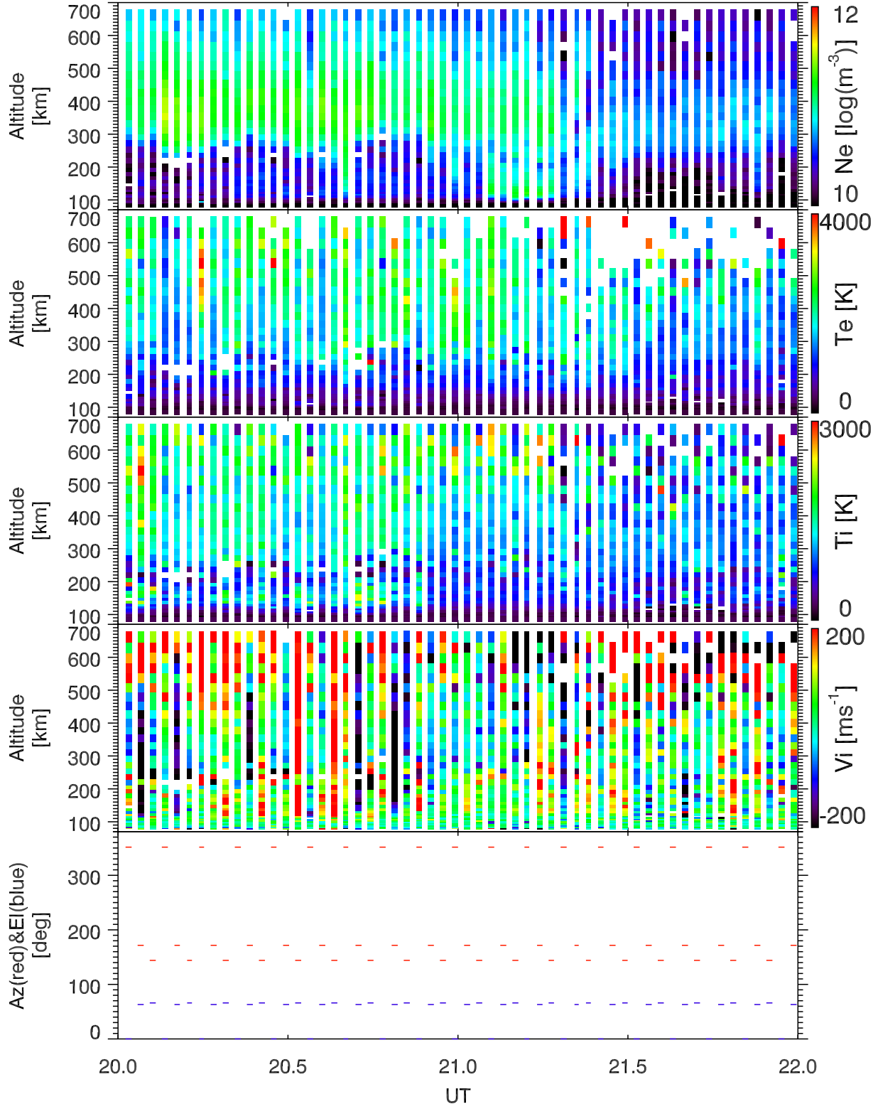
EISCAT 2003-11-18_20_22UT_steffe_ant@32m.
