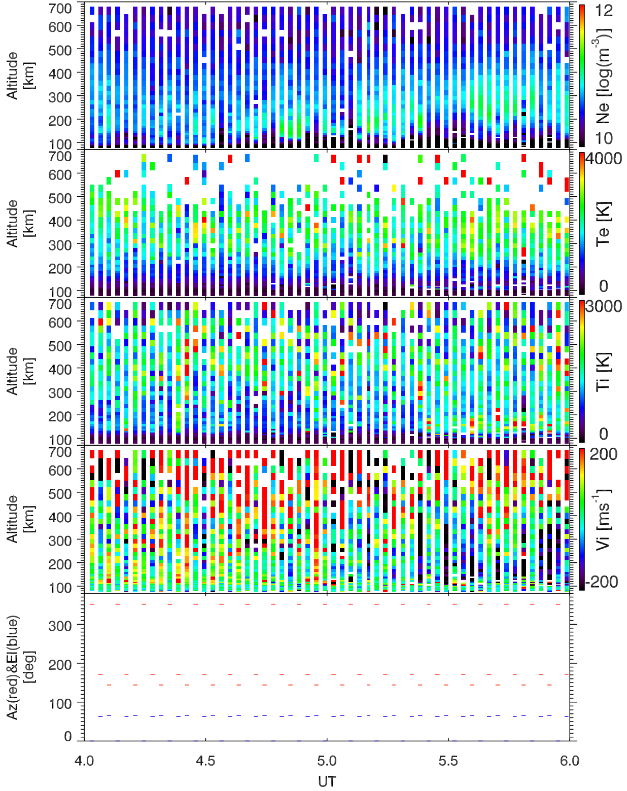
EISCAT 2003-11-19_04_06UT_steffe_ant@32m.
