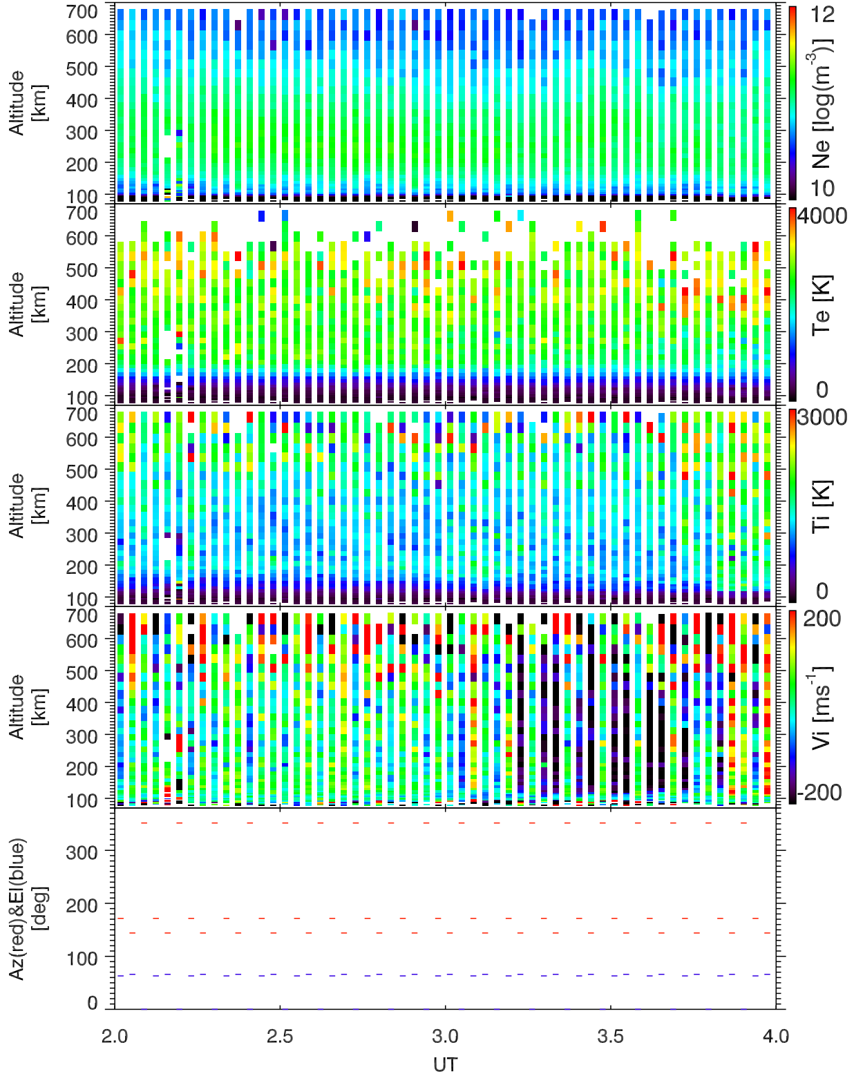
EISCAT 2004-06-06_02_04UT_steffe_ant@32m.
