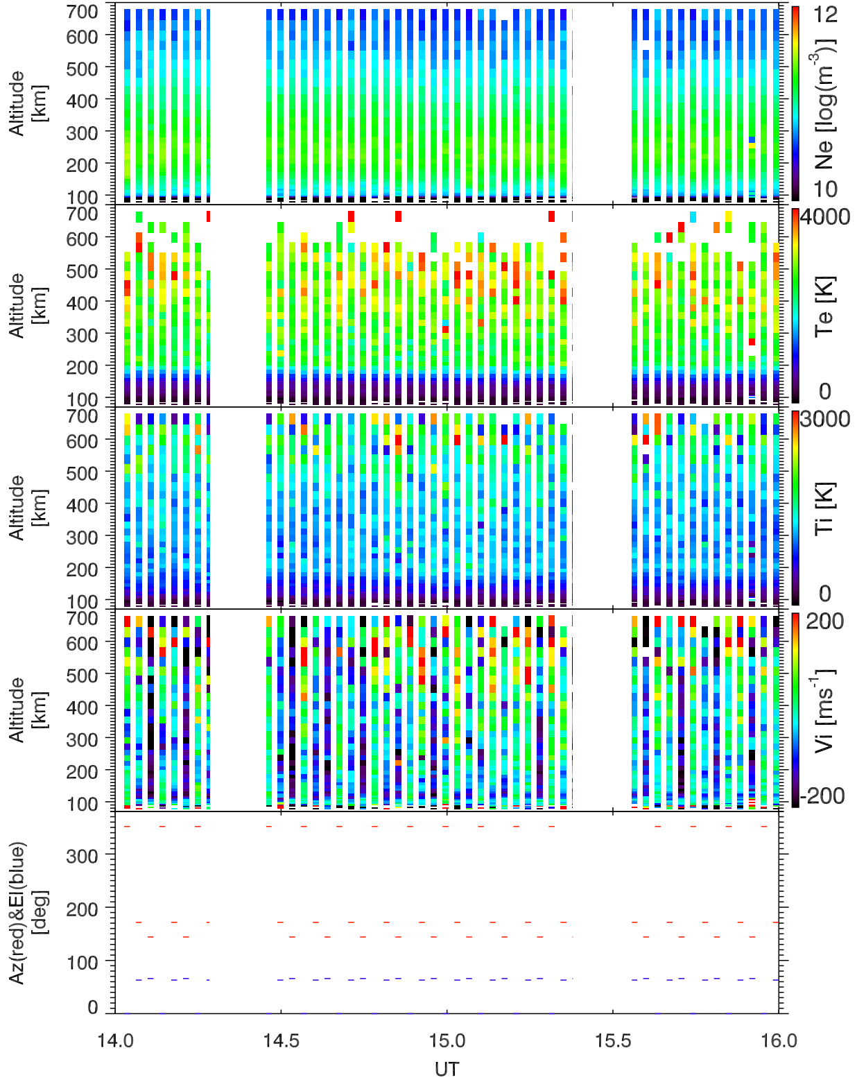
EISCAT 2004-06-08_14_16UT_steffe_ant@32m.
